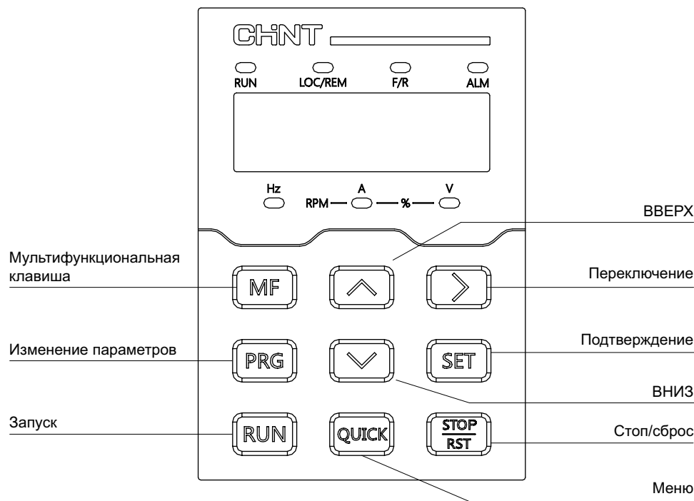
Рис. 7.7.1 LED-панель
