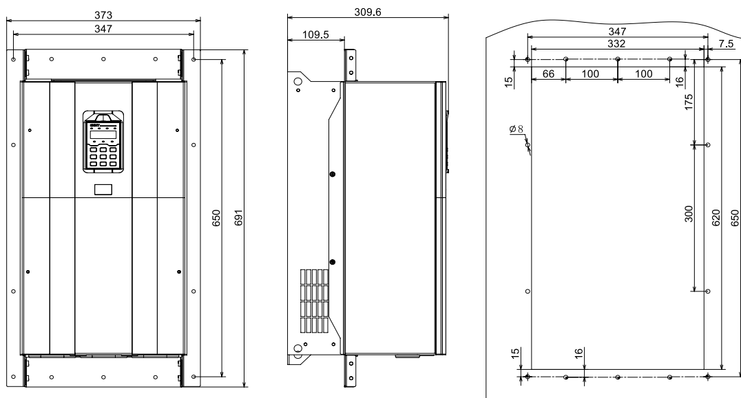
Рис. 6.2.6 Комплект фланцевого монтажа для типоразмера T7
