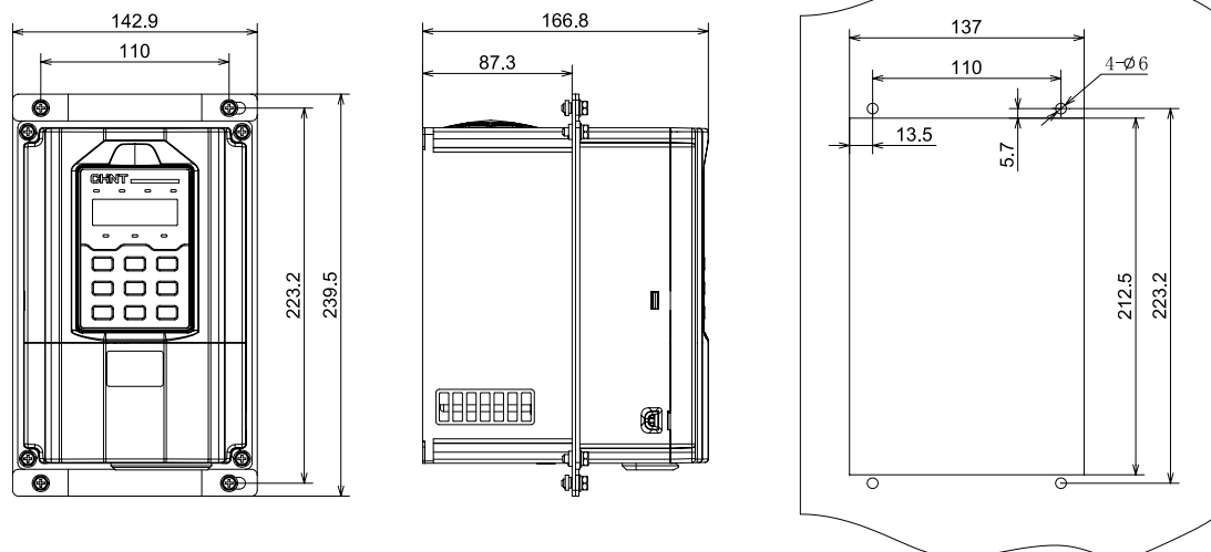
Рис. 6.2.1 Комплект фланцевого монтажа для типоразмера T2
